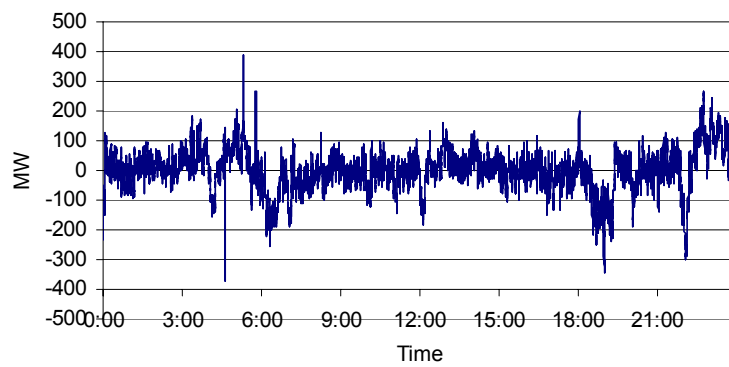
ISO-ACE, 1-Oct-2003
