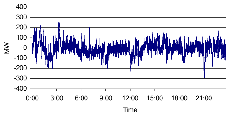
ISO-ACE, 18-Oct-2003
