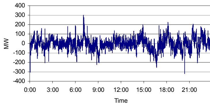
ISO-ACE, 12-Apr-2003
